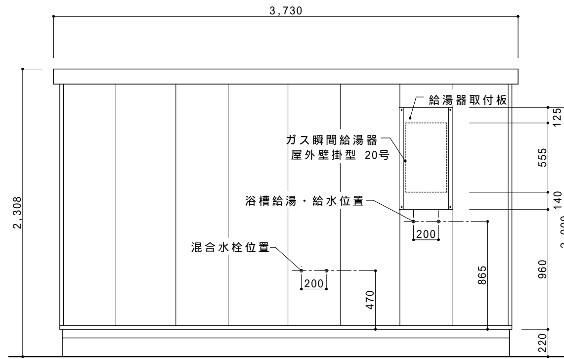
断面図 S=1/30
