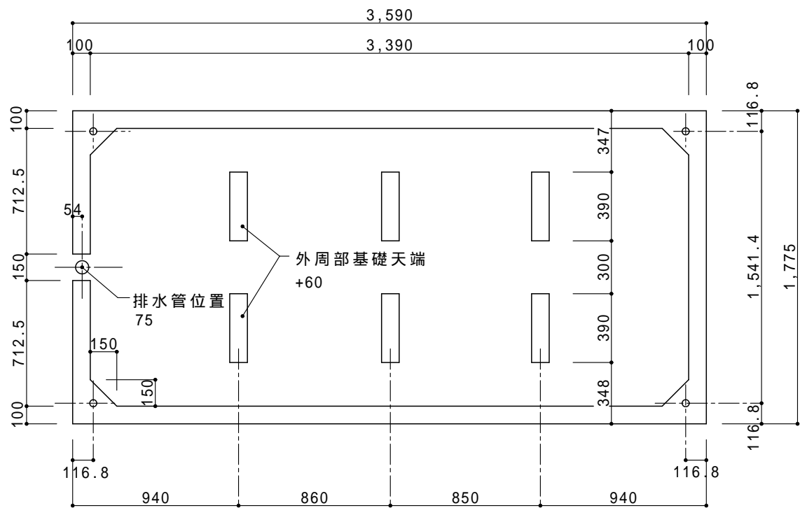
基礎参考図 S=1/30
