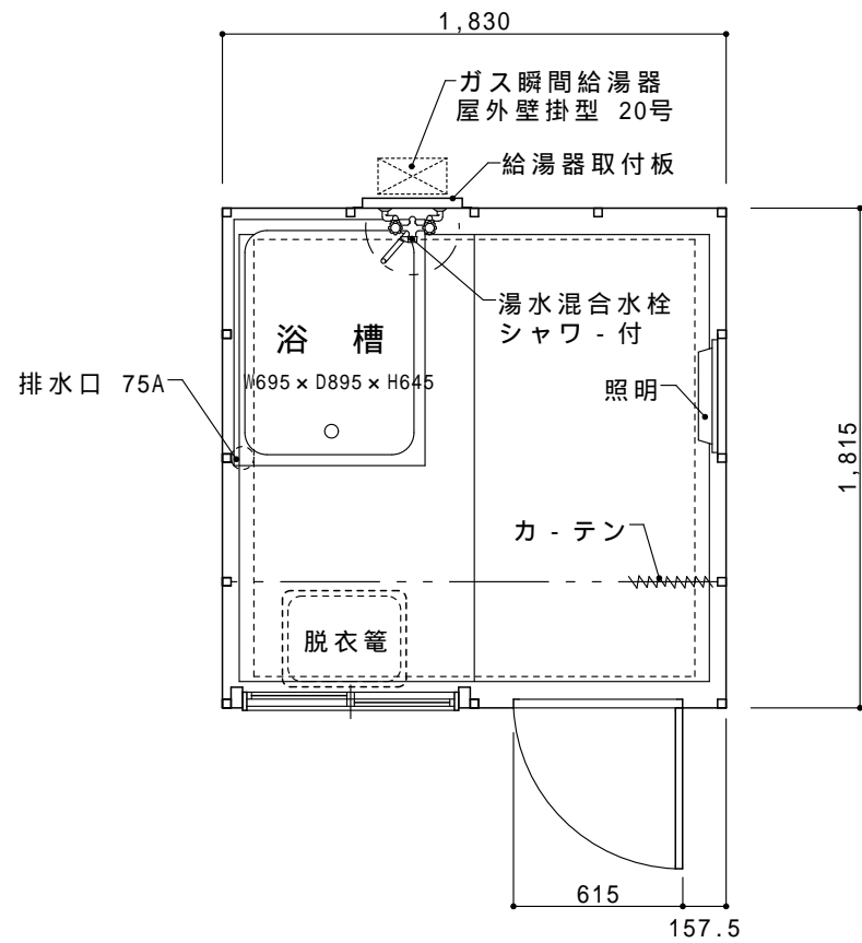
平面図 S=1/30
