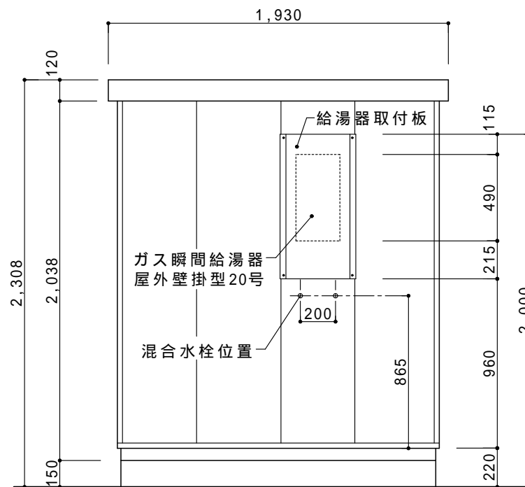
断面図 S=1/30
